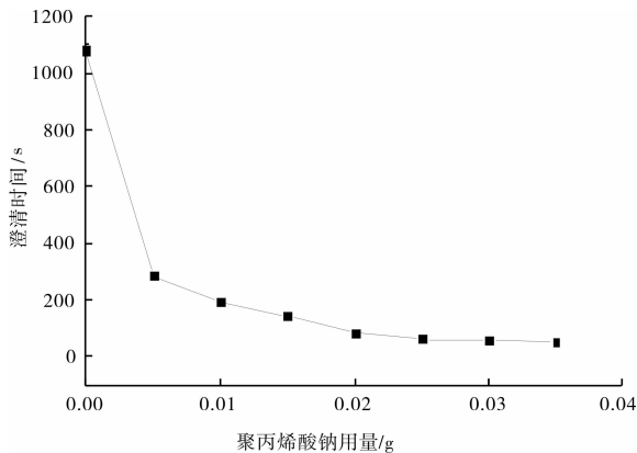
图4 聚丙烯酸钠用量与澄清时间的关系
