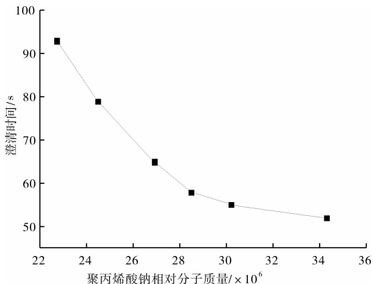
图3 聚丙烯酸钠相对分子质量与絮凝时间的关系
