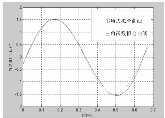
图7 绕组2电压变化的多项式拟合曲线与三角函数拟合曲线
