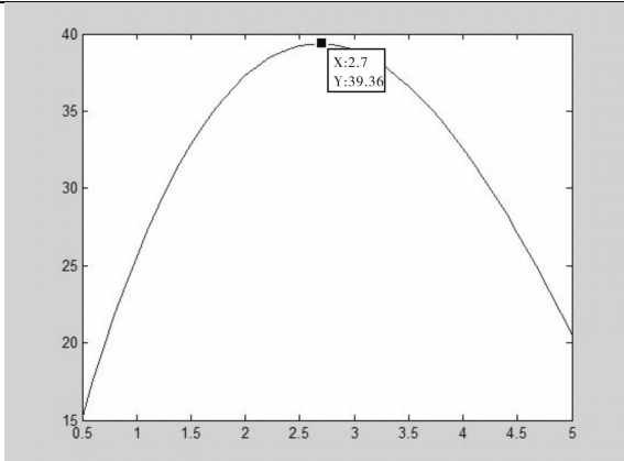
图 4 水轮转速与输出功率的关系图
