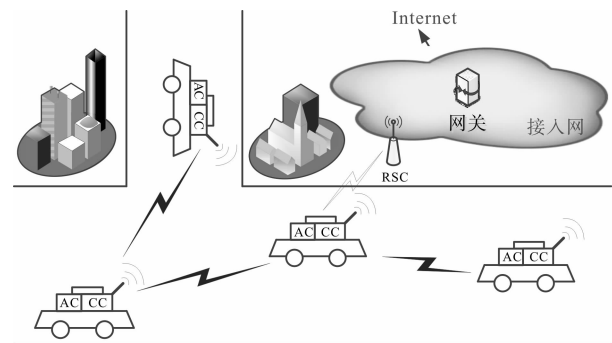
图1 VANET基本结构图
