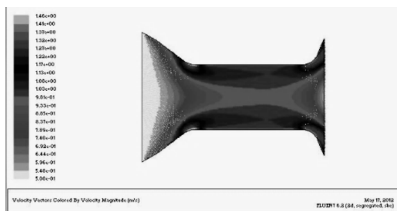
图 1 2D 导流罩模型水流速度分布图
