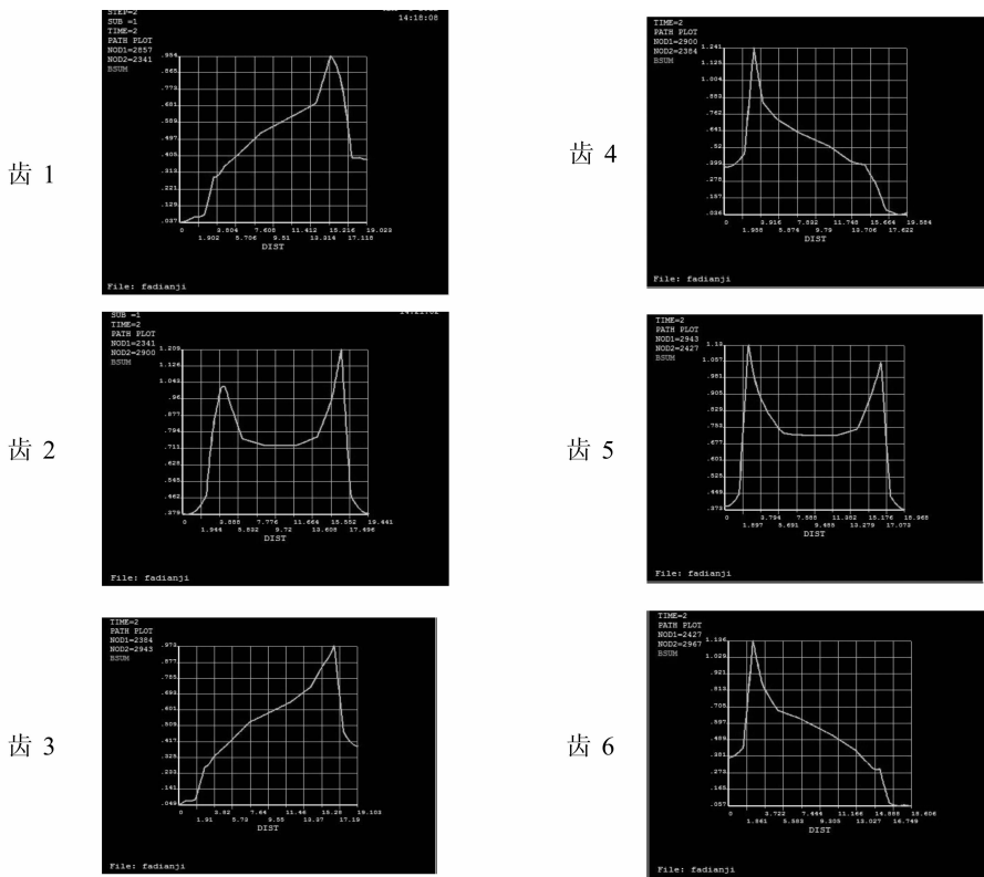
图 5 \theta = 0^\circ 时齿 1 至齿 6 间的气隙磁通量大小变化图
