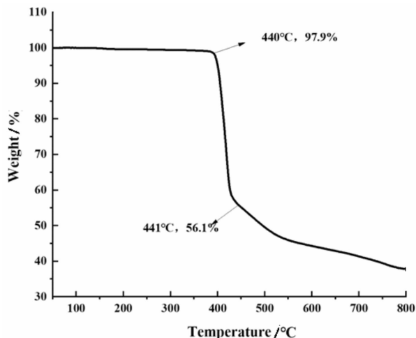
图10 配合物 Z6 的 TGA 图
