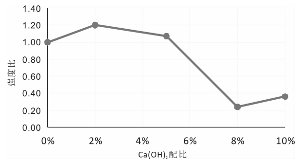
图4 \text{Ca}(\text{OH})_2 掺量对黄河淤泥生态砌块强度的影响
