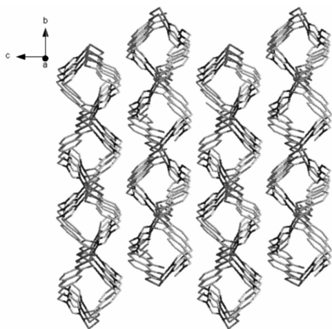
图4 配合物 Z6 沿 a 轴方向的三维(3D)平面图
