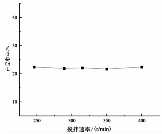
图 7 搅拌速率对收率的影响
