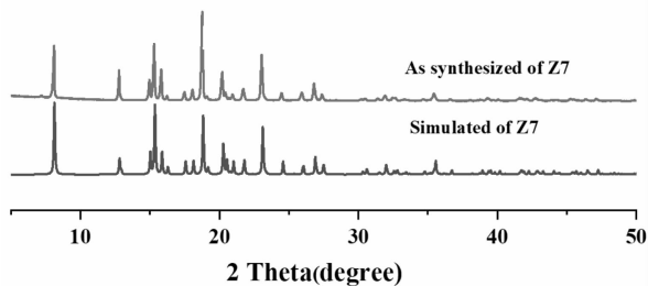
图9 配合物 Z7 的 X-射线粉末衍射图
