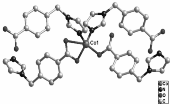
图2 配合物 Z6 的金属配位环境图
