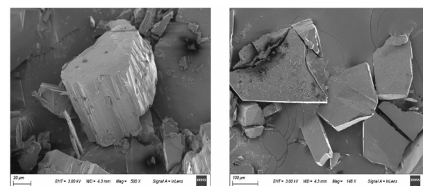
图 14 配合物 Z7 的 SEM 图
