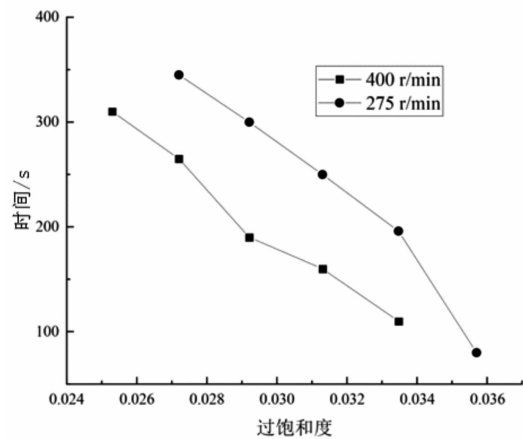
图4 搅拌速率对诱导期的影响
