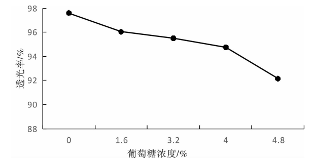
图 4 不同葡萄糖浓度对乳清蛋白 - 葡萄糖可食性膜透光率的影响
