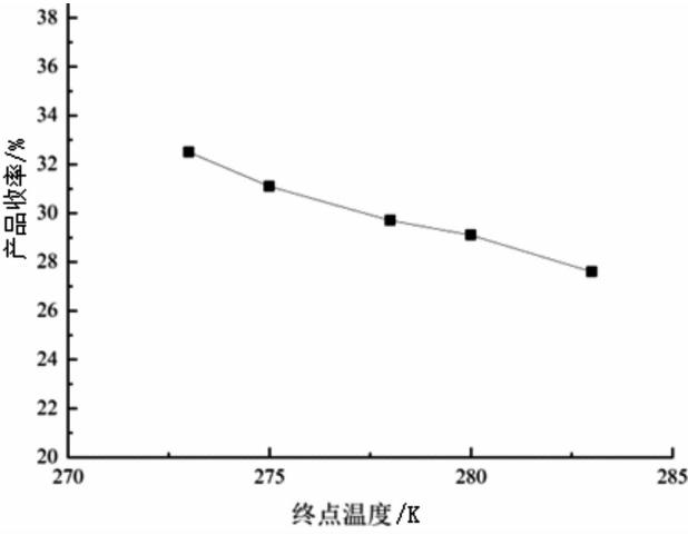
图 9 终点温度对收率的影响
