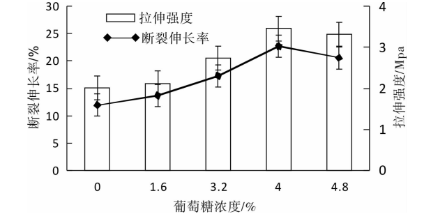
图 5 不同葡萄糖浓度对乳清蛋白 - 葡萄糖可食性膜机械性能的影响
