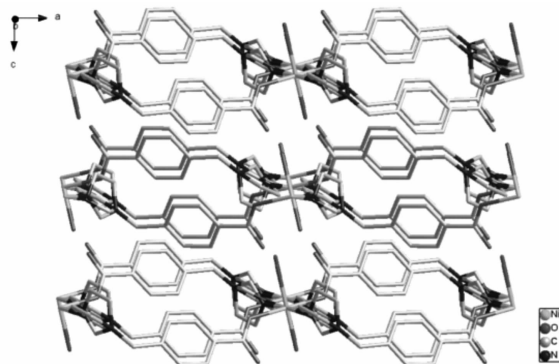
图7 配合物 Z7 沿 b 轴方向的三维(3D)堆积图
