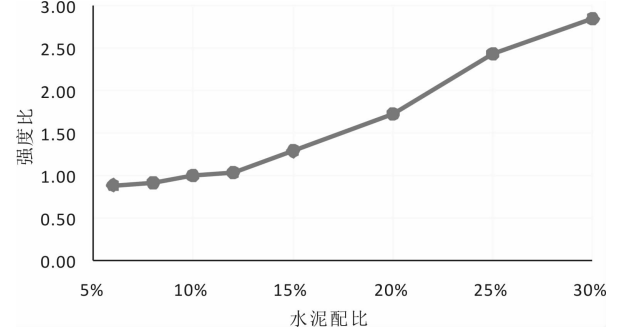
图 3 水泥掺量黄河淤泥试块抗压强度
