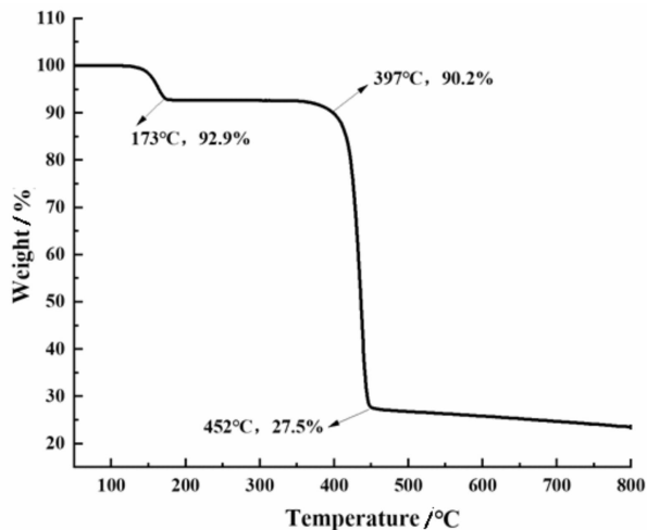
图11 配合物 Z7 的 TGA 图
