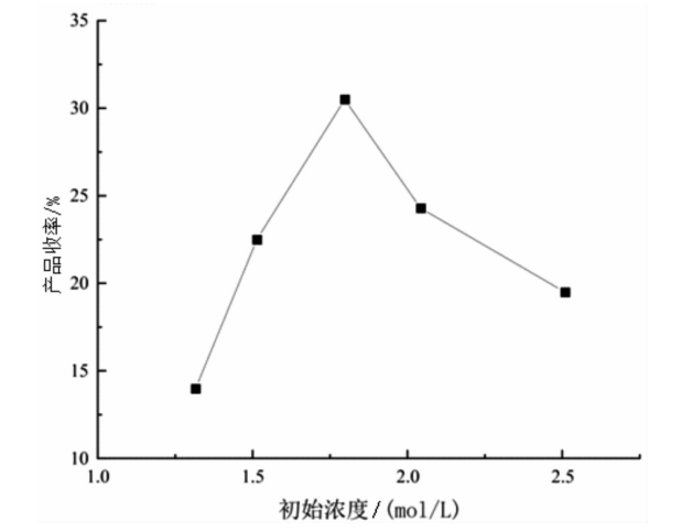
图 8 初始浓度对收率的影响
