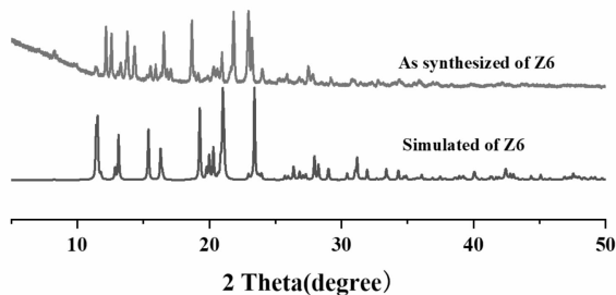
图8 配合物 Z6 的 X - 射线粉末衍射图
