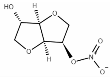
图1 5-单硝酸异山梨酯结构式
