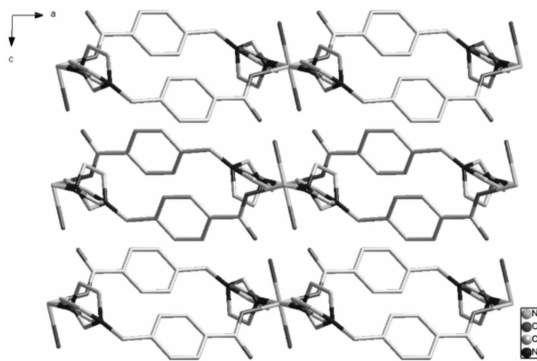
图6 配合物 Z7 沿 b 轴方向的二维(2D)平面图
