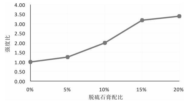
图5 脱硫石膏掺量对黄河淤泥生态砌块强度的影响
