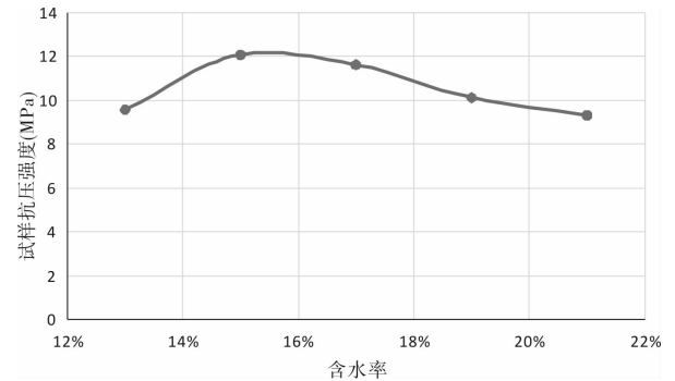
图 2 试样含水率和抗压强度关系图
