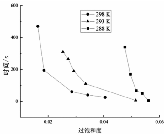
图5 温度对诱导期的影响
