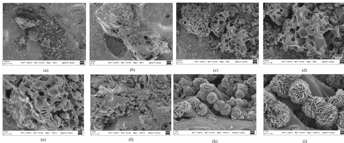
图 13 800 ^{\circ}\text{C} 高温灼烧后的 Z6 SEM 图
