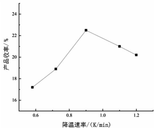
图6 降温速率对收率的影响
