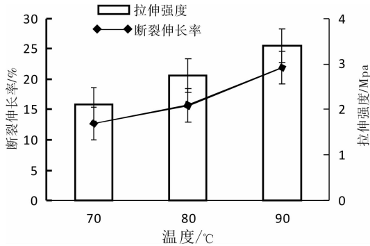
图 2 温度对乳清蛋白 - 葡萄糖可食性膜机械性能的影响
