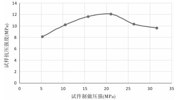
图 1 试样制作加压强度和试样抗压试验强度关系图
