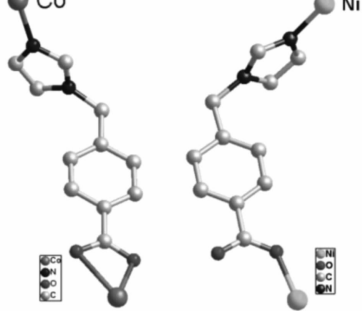
图 1 配体在配合物 Z6 和 Z7 中所呈现的配位模式
