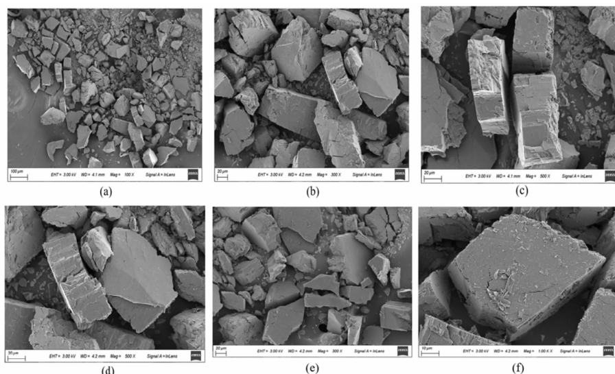
图 15 800 ^{\circ}\text{C} 高温灼烧后的 Z7 SEM 图
