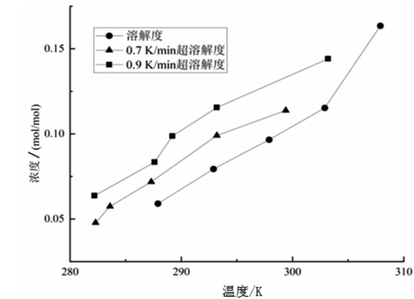
图2 降温速率对介稳区宽度的影响
