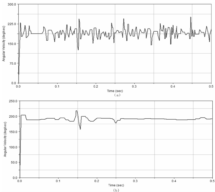
图 5 行星轮公转角速度
