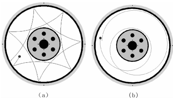
图7 工件相对于研磨盘运动轨迹
