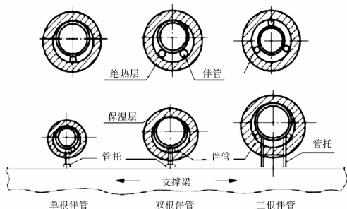
图3 蒸汽伴管的标准设置
