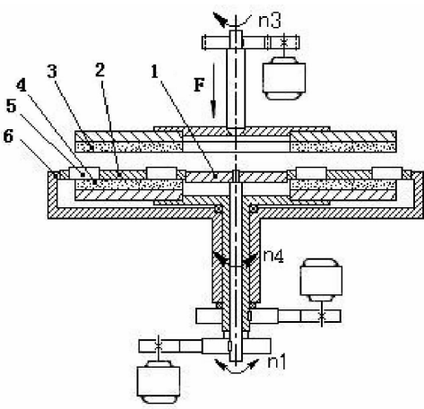
图2 研磨机运动原理图
