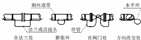
图4 蒸汽伴管膨胀弯
