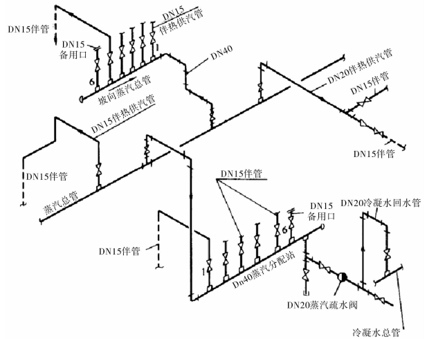
图2 蒸汽分配站和供汽管的布置
