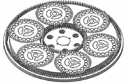
图3 研磨机三维模型
