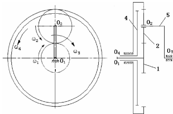
图 1 研磨机结构及运动示意图
