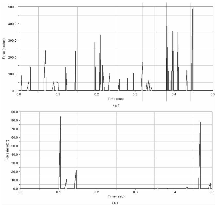
图 6 行星轮与内齿圈接触力
