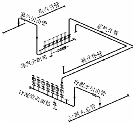
图1 蒸汽伴热管道系统图
