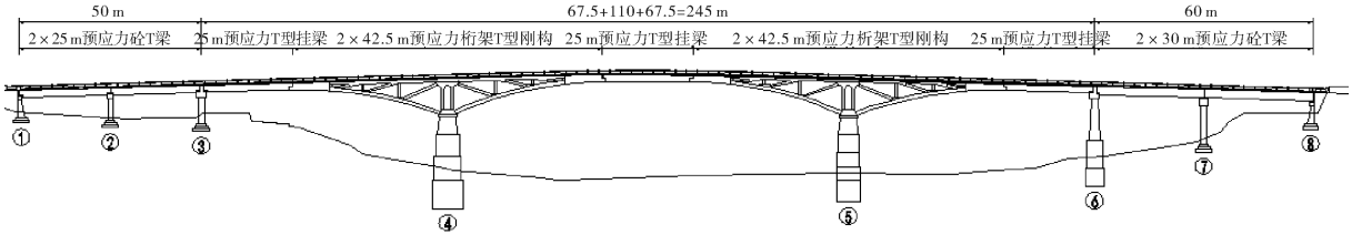
图1 既有桥桥型布置图
