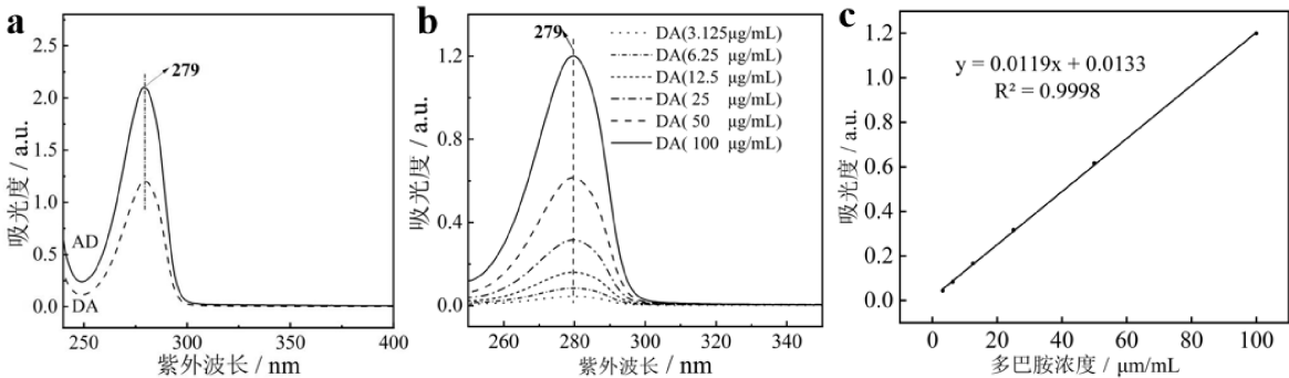
图3 (a) 多巴胺和海藻酸钠-多巴胺样品的紫外可见光吸收光谱图; (b) 不同浓度的多巴胺溶液的紫外可见光光谱; (c) 多巴胺溶液浓度-吸收强度标准曲线
