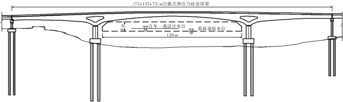
图 4 主桥设计方案
