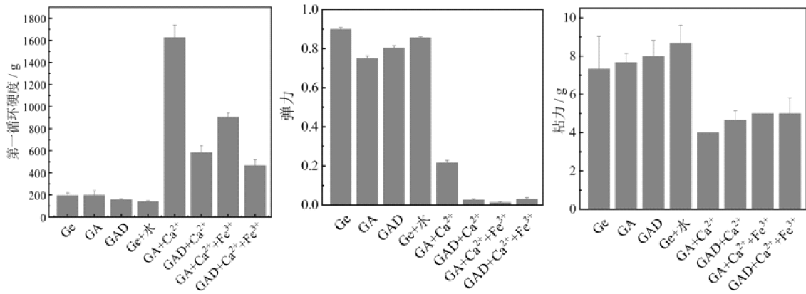
图5 海藻酸钠-多巴胺缀合物和金属离子对明胶水凝胶样品的质构性能影响
