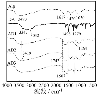
图 1 Alg、DA 和 AD 的红外光谱图
