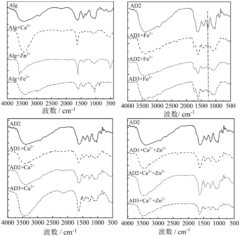
图4 海藻酸钠-多巴胺与离子相互作用的红外光谱
