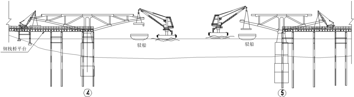
图3 主桥 T 构拆除示意图
