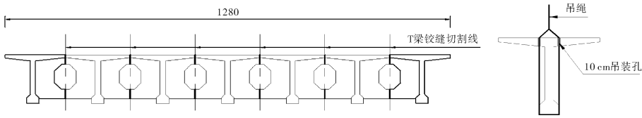
图2 引桥 T 梁拆除示意图
