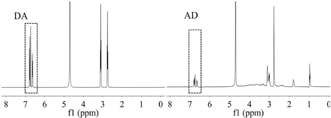
图 2 DA 和 AD 的 1 H-NMR 谱图
